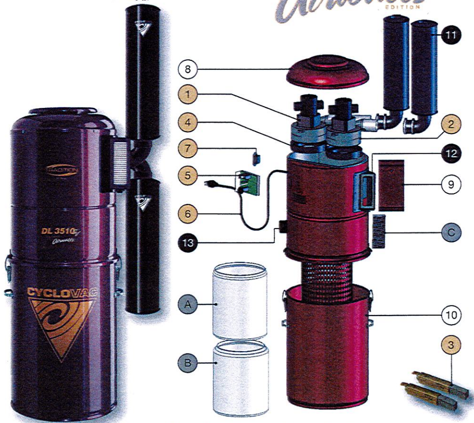
Parts list • Liste de pièces • Lista de piezas
